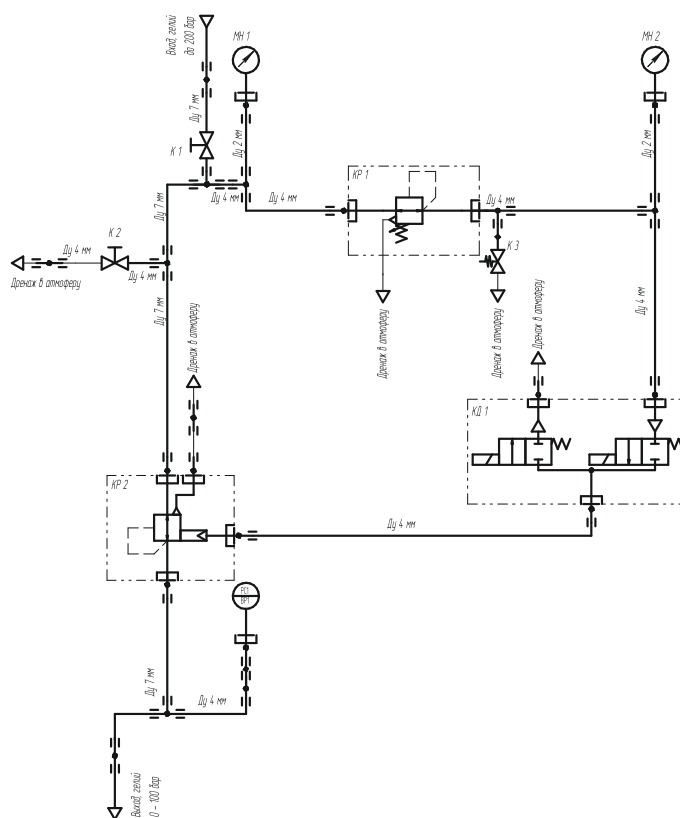
Пример принципиальной схемы работы автоматизированного модуля контроля давления.
