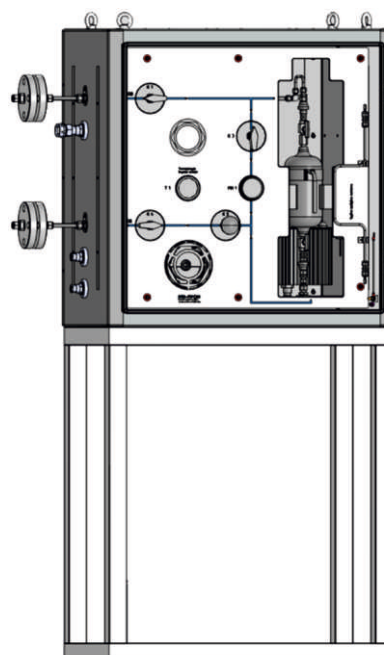
Пример системы отбора проб, разработанной нашими специалистами. Устройство пробоотбора обеспечивает возможность отбора проб агрессивной среды из магистрали.
