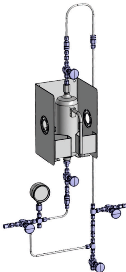
Пример системы отбора проб, разработанной нашими специалистами. Устройство пробоотбора обеспечивает возможность отбора проб агрессивной среды из магистрали.
