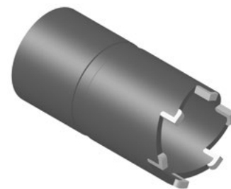
Фрезер типа 1ФК
